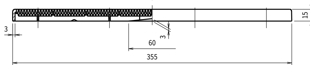
B-B断面図
